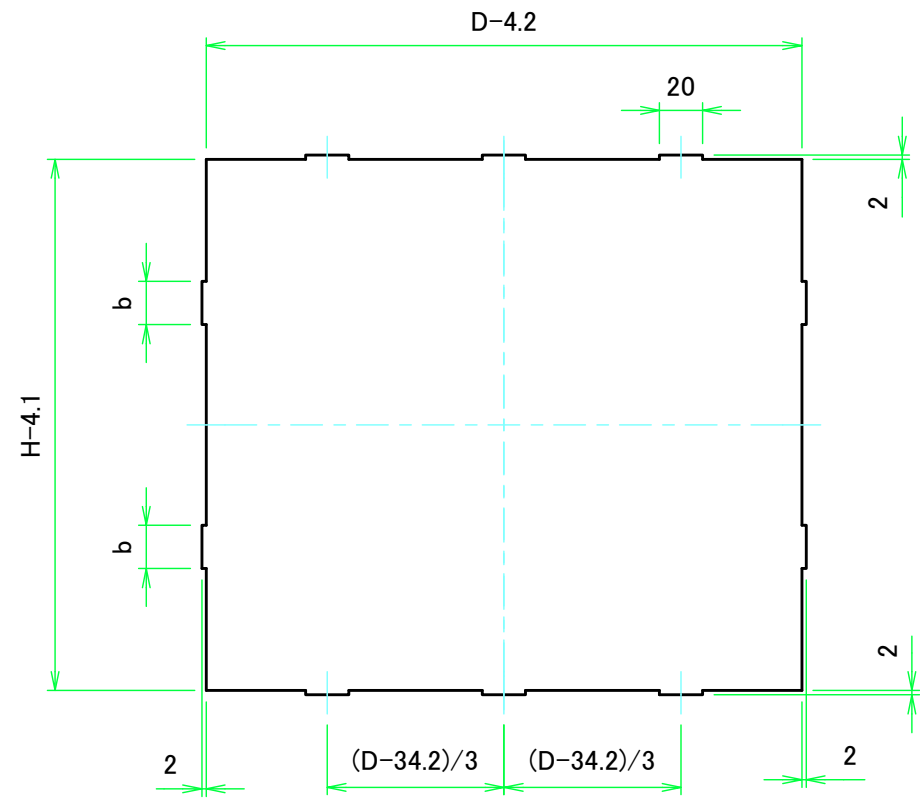
Dパネル1表面 / D panel 1 Frontside
